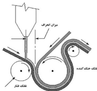
شکل ۵ فرایند تهیه فیلم به روش چندلاسازی اکسترودر.
